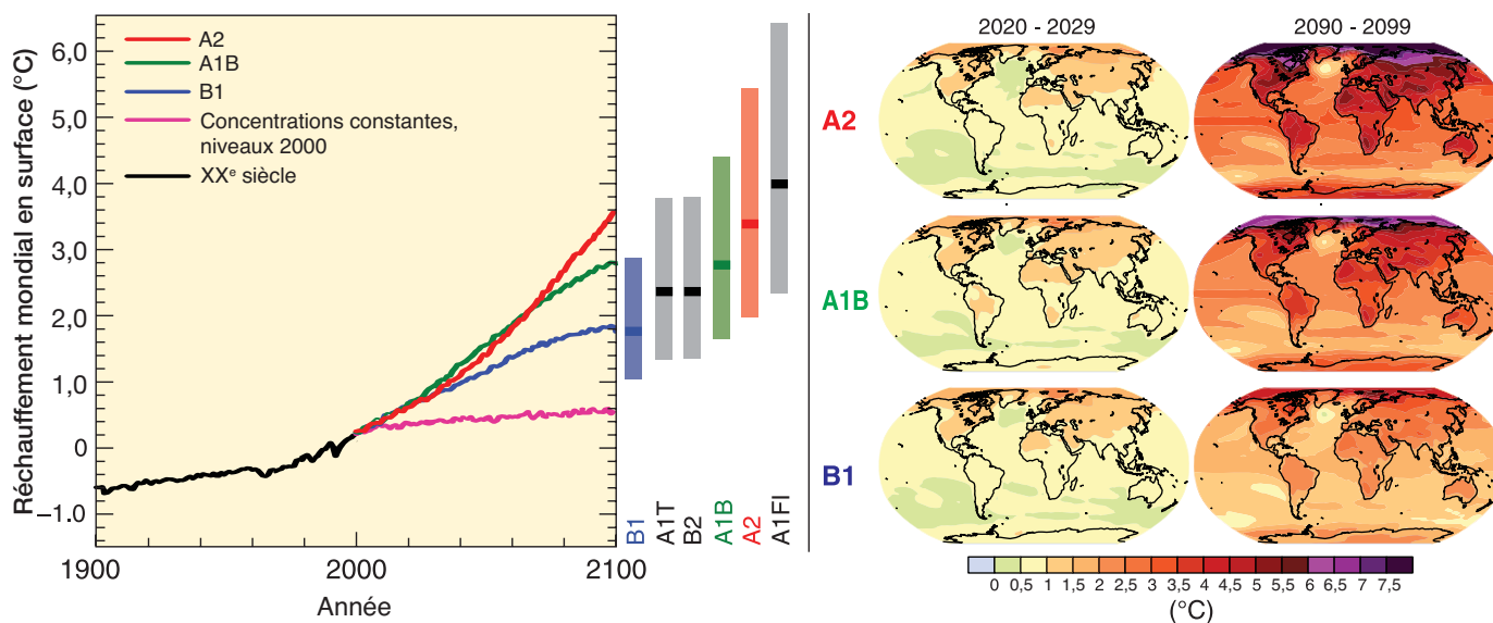
Figure 3.2. À gauche : Les courbes en trait plein correspondent aux moyennes multimodèles du réchauffement en surface (par rapport à la période 1980-1999) pour les scénarios A2, A1B et B1 du SRES, dans la continuité des simulations relatives au XX e siècle. La courbe orange correspond au cas où les concentrations se maintiendraient aux niveaux de 2000. Les barres au milieu de la figure indiquent les valeurs les plus probables (zone foncée) et les fourchettes probables selon les six scénarios SRES de référence pour la période 2090-2099 par rapport à 1980-1999. Ces valeurs et ces fourchettes tiennent compte des projections établies à l'aide des modèles de la circulation générale couplés atmosphère-océan (MCGAO) (partie gauche de la figure) ainsi que des résultats d'une hiérarchie de modèles indépendants et des contraintes liées à l'observation. À droite : Évolution projetée de la température en surface pour le début et la fin du XXI e siècle par rapport à la période 1980-1999, selon les projections moyennes obtenues à l'aide de plusieurs modèles MCGAO pour les scénarios A2 (en haut), A1B (au milieu) et B1 (en bas) du SRES, pour les décennies 2020-2029 (à gauche) et 2090-2099 (à droite). {GT I 10.4, 10.8 ; figures 10.28, 10.29, RiD}
